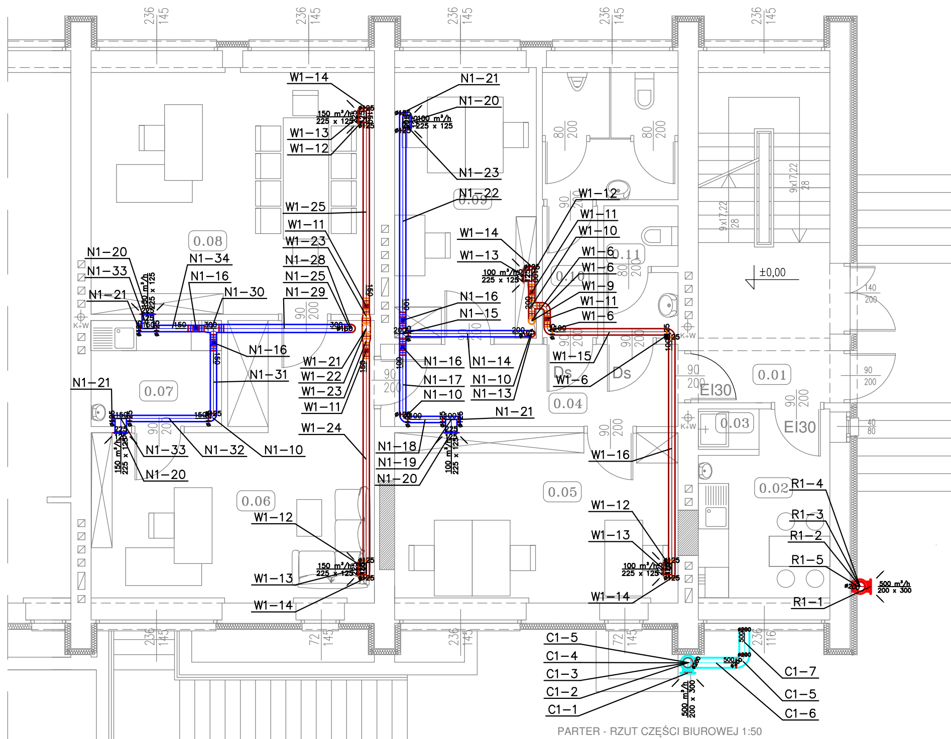
PARTER - RZUT CZĘŚCI BIUROWEJ 1:50
